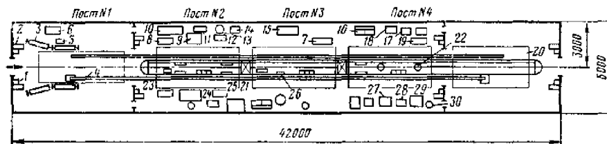
Рисунок Б.6 – Схема технологической планировки поточной линии ТО-2:
